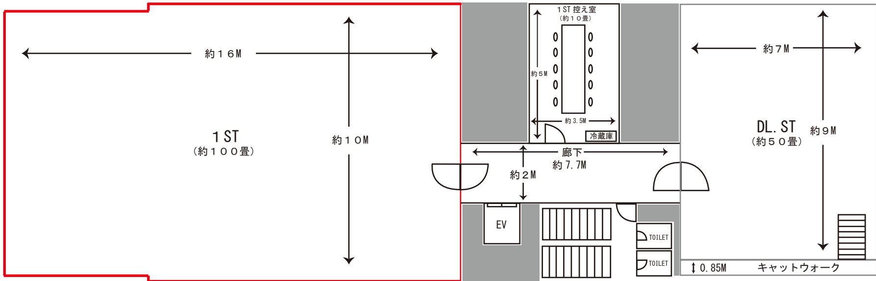
2F フロア図面
